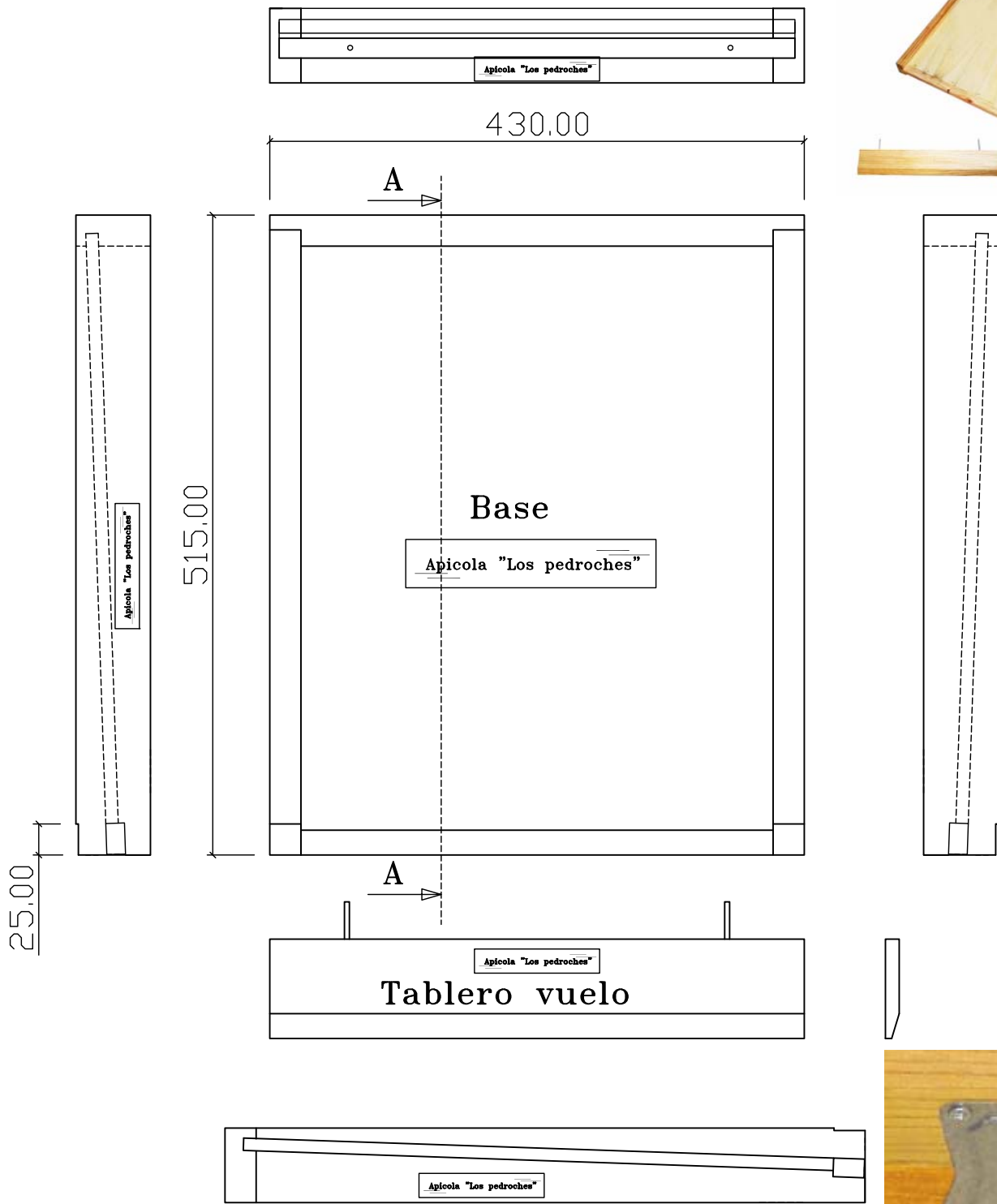
Seccion A-A
