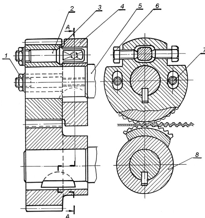
Fig.8 esquema de rotación de rodillo superior alrededor de su eje.
