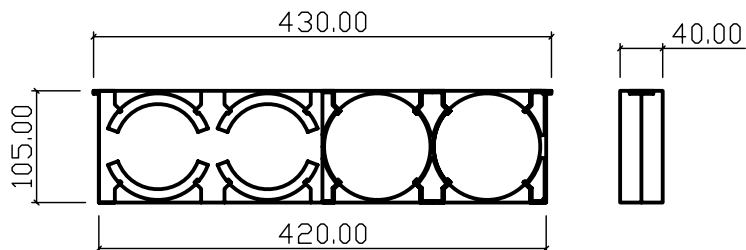
VISTA A-A
