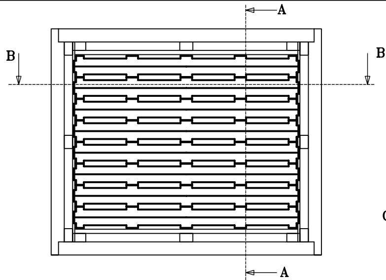
DETALLE ALZA MODIFICADA
