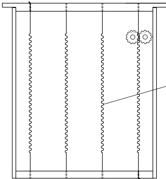
CUADRO LAYENS CON ALAMBRE DESPUES DE PASAR EL TENSOR
